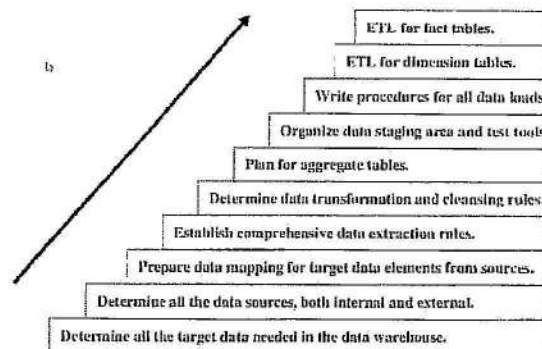
ภาพประกอบที่ 3 รูปแสดงขั้นตอนการทำ ETL
