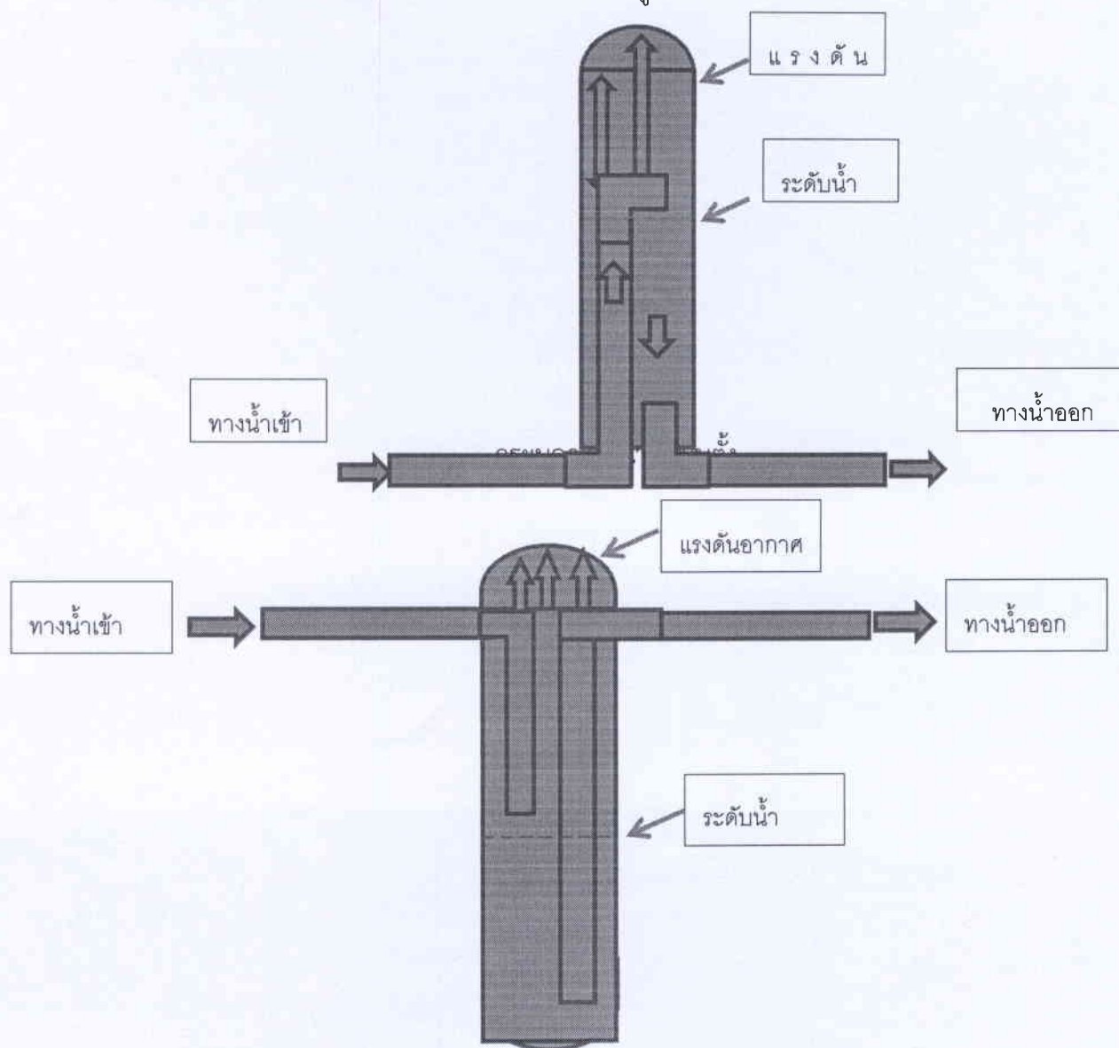
ภาพการทำงานของแอร์แวแบบฝังลงในพื้นดิน
