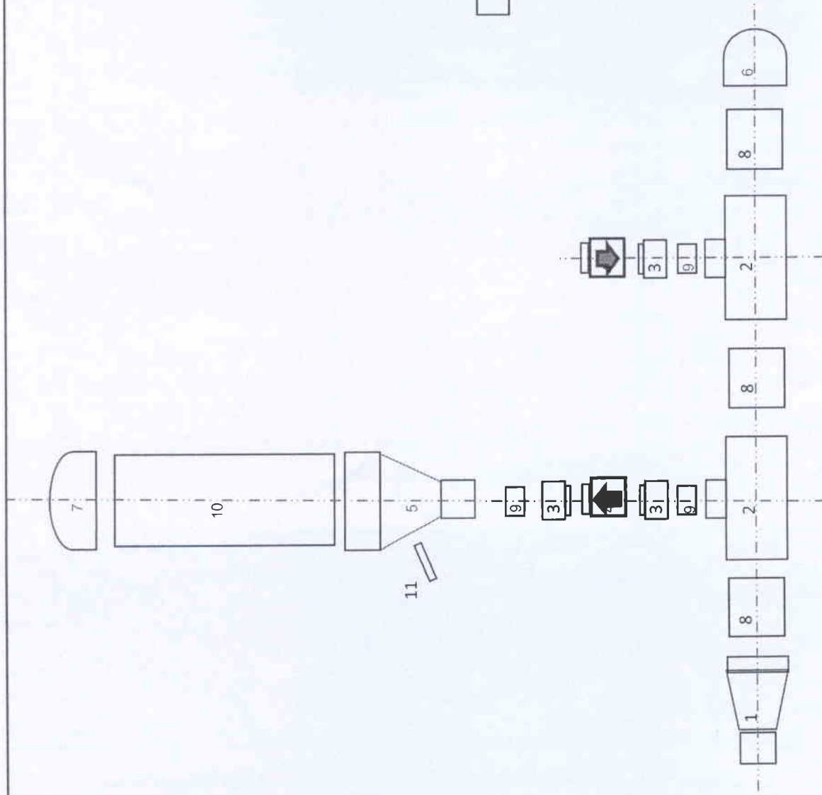
ภาพแยกส่วนเครื่องตะบันน้ำ
